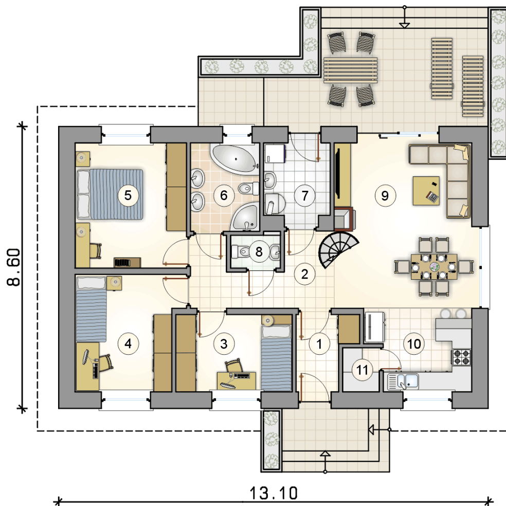
RZUT PARTERU
