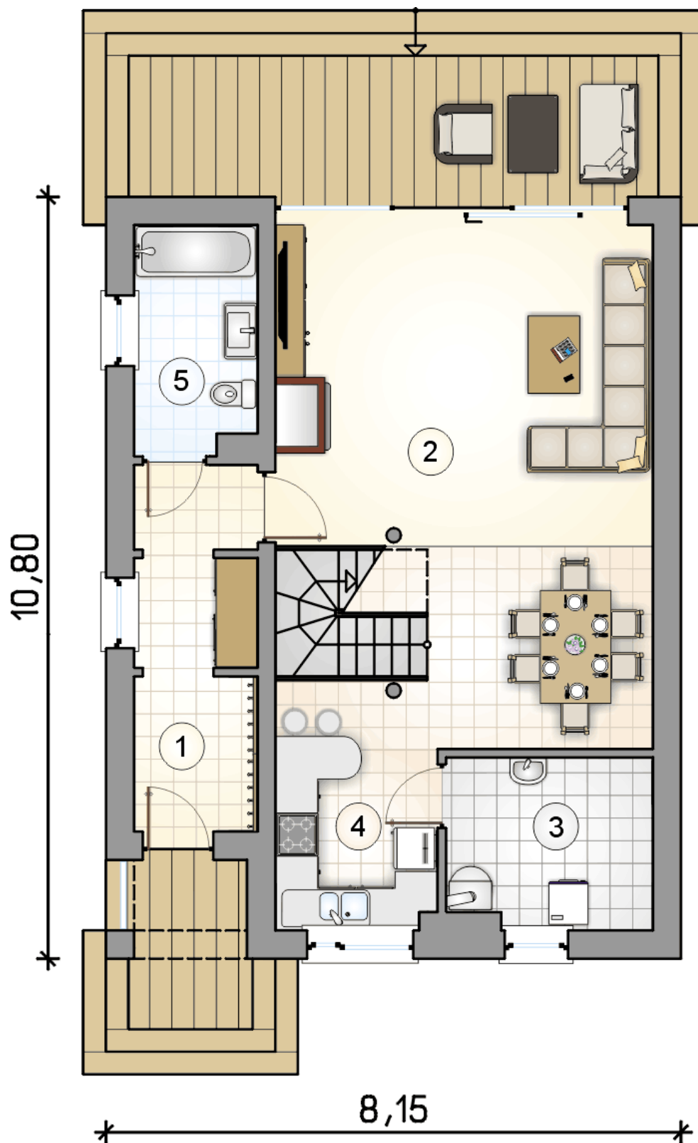
RZUT PARTERU
