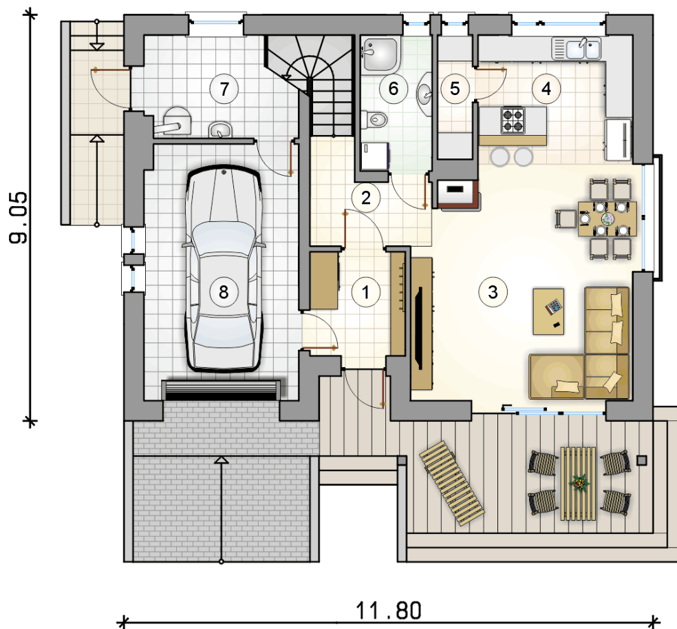
RZUT PARTERU
