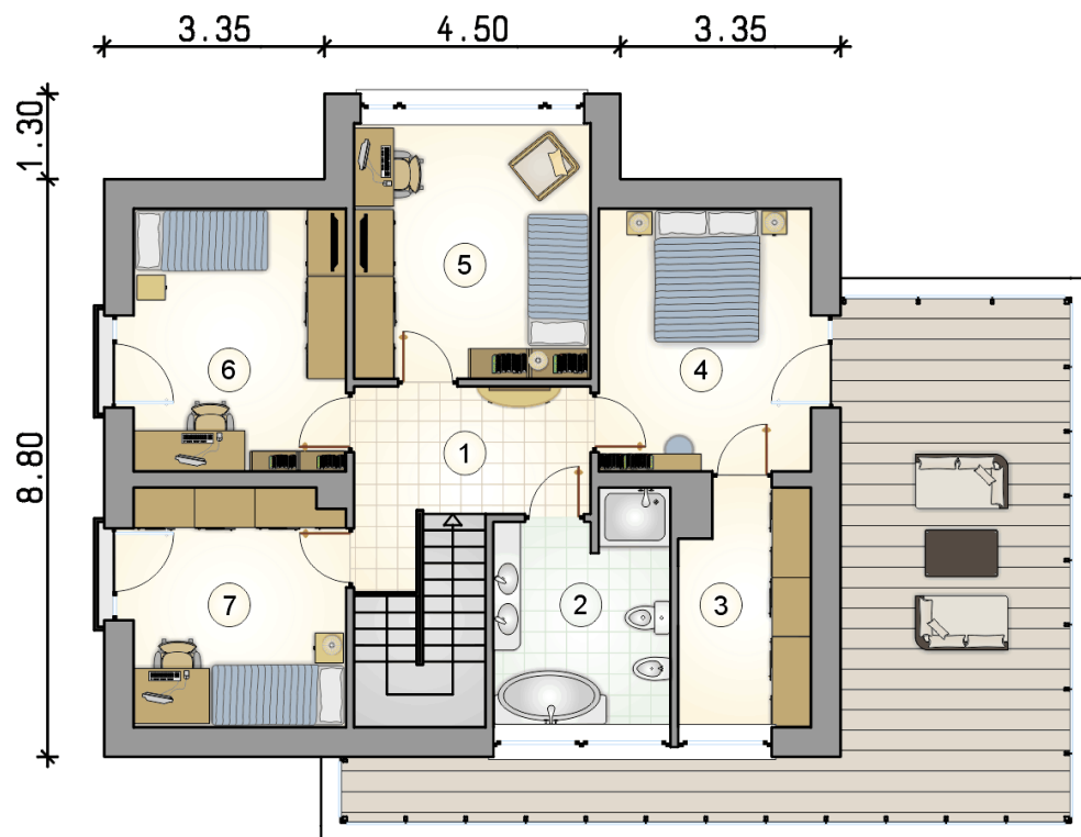
RZUT PIĘTRA
