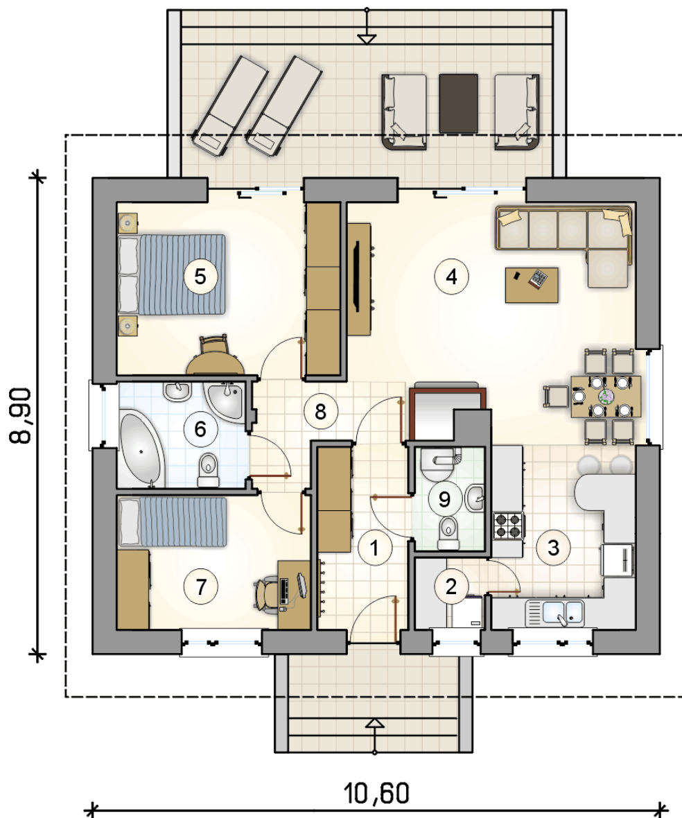
RZUT PARTERU
