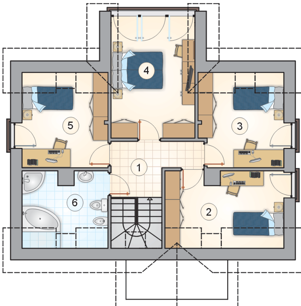
RZUT PODDASZA
